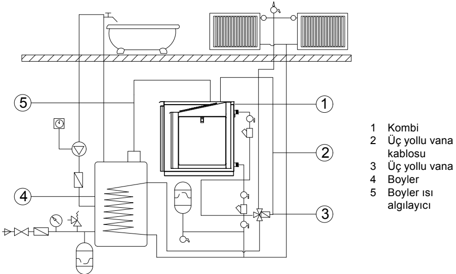
Elektrikli kombi, boyler ve radyatör bağlantı şeması.
